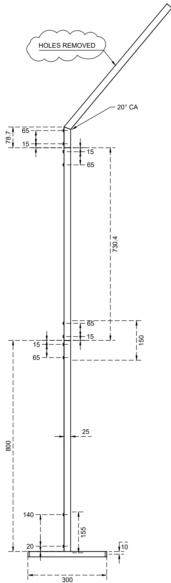
END ELEVATION
